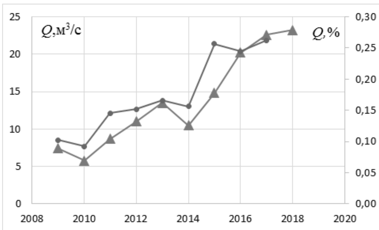
Рисунок 1. Многолетняя динамика среднегодовых расходов воды пр. Шароновка (пост Ганюшкино, нижняя линия) и его стоковой доли от руслового стока р. Волги (пост Верхнее Лебяжье), по данным Казгидромета
