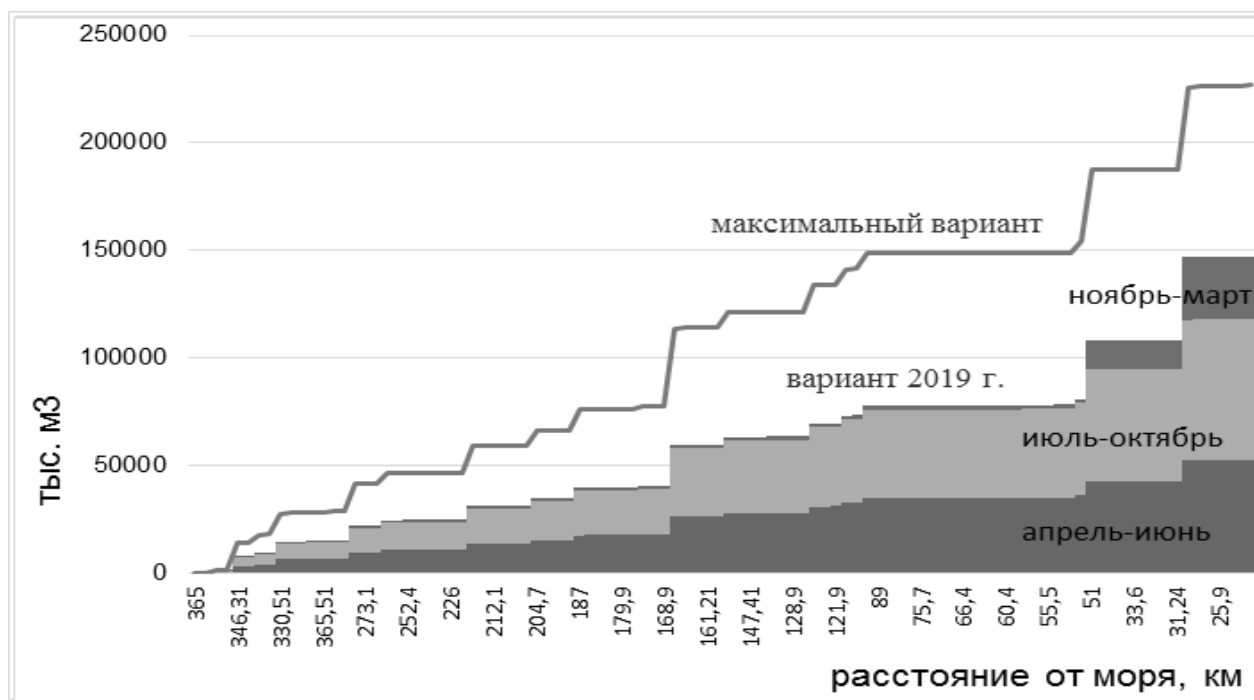
Рисунок 3. Нарастание годовых объемов забора воды из р. Урал в пределах Атырауской обл. с разделением на сезоны для варианта 2019 г.
