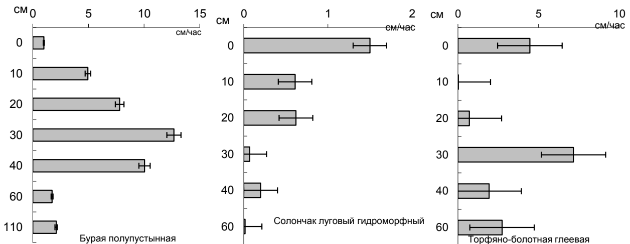
Рисунок 2. Коэффициенты фильтрации почв участка № 1
