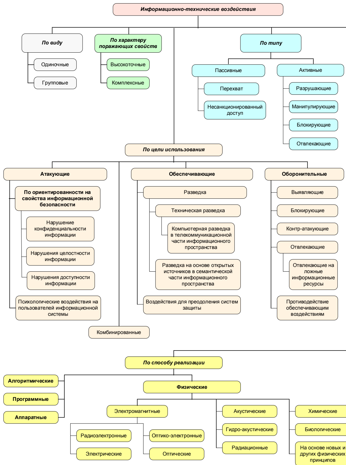
Рисунок 1. Классификация ИТВ, предназначенных для тестирования объектов КИИ [Макаренко 2018б]
