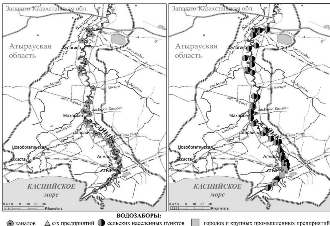
Рисунок 2. Карта-схема каналов, размещения и назначения водозаборных сооружений по длине р.Урал (по состоянию на 2019 г.)
