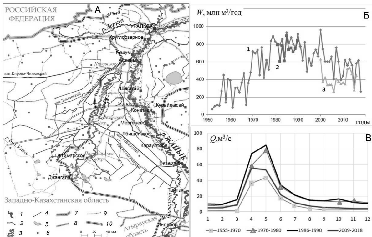
Рисунок 1. Урало-Кушумская ООС (А), многолетние (Б) и внутригодовые (В) показатели забора воды Кушумским каналом. Условные обозначения: (А) 1 – пойменно-русловой комплекс нижнего Урала (Жайык), 2 – другие реки, 3 – Кушумский канал с водохранилищами, 4 – каналы, 5 – водоемы, 6 – населенные пункты, 7 – госграница, 8 и 9 – границы областей и районов, 10 – граница бассейна р.Урал; (Б) по данным гидрологических ежегодников и Казгидромета (1 и 2), Западно-Казахстанского филиала РГП «Казводхоз» (3)
